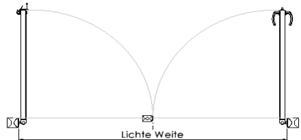
Öffnungsrichtung – Schwenkbereich 90°
