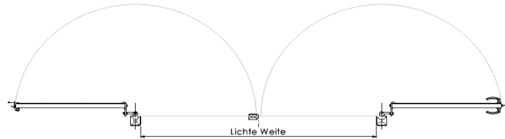
Öffnungsrichtung – Schwenkbereich 180°
